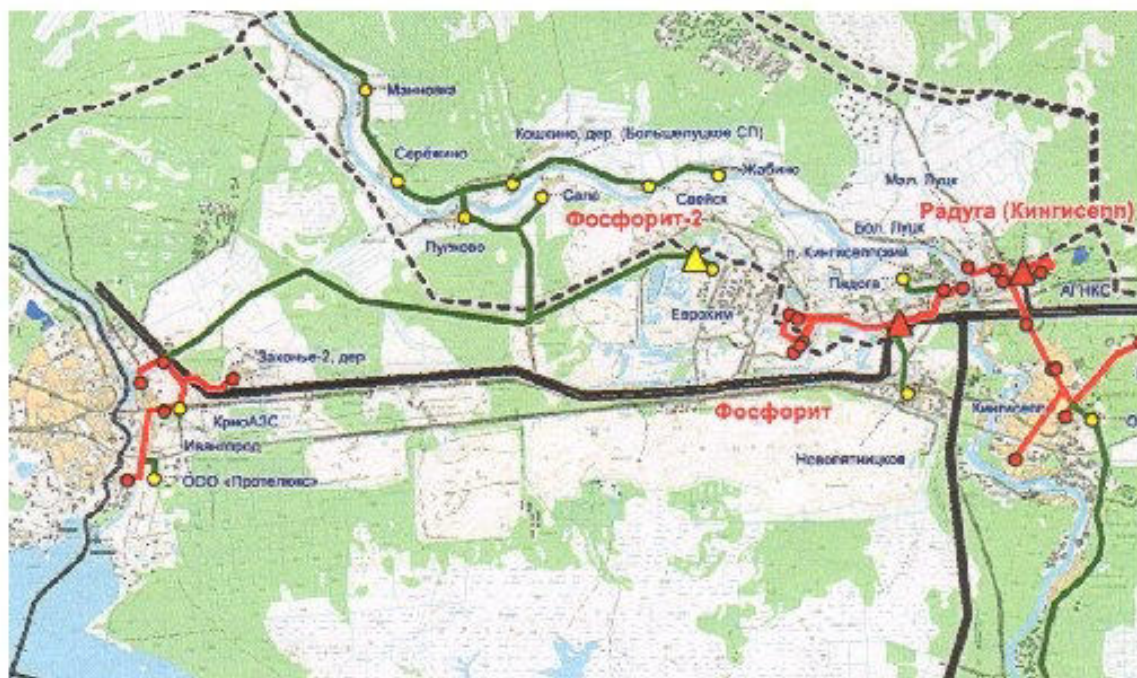
Рисунок П.1 – Схема газоснабжения и газификации МО «Большелуцкое сельское поселение»
