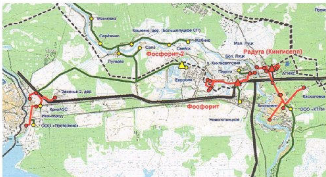
Рисунок П.1 – Схема газоснабжения и газификации МО «Большелуцкое сельское поселение»
